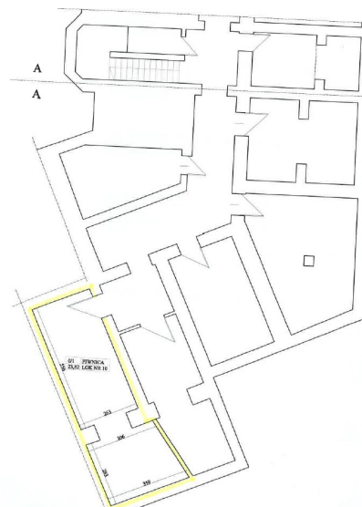
Rzut piwnicy
