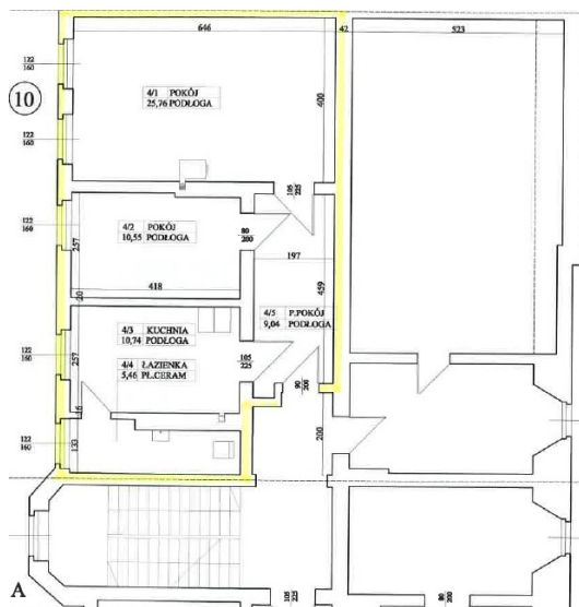
Rzut 3-go piętra
